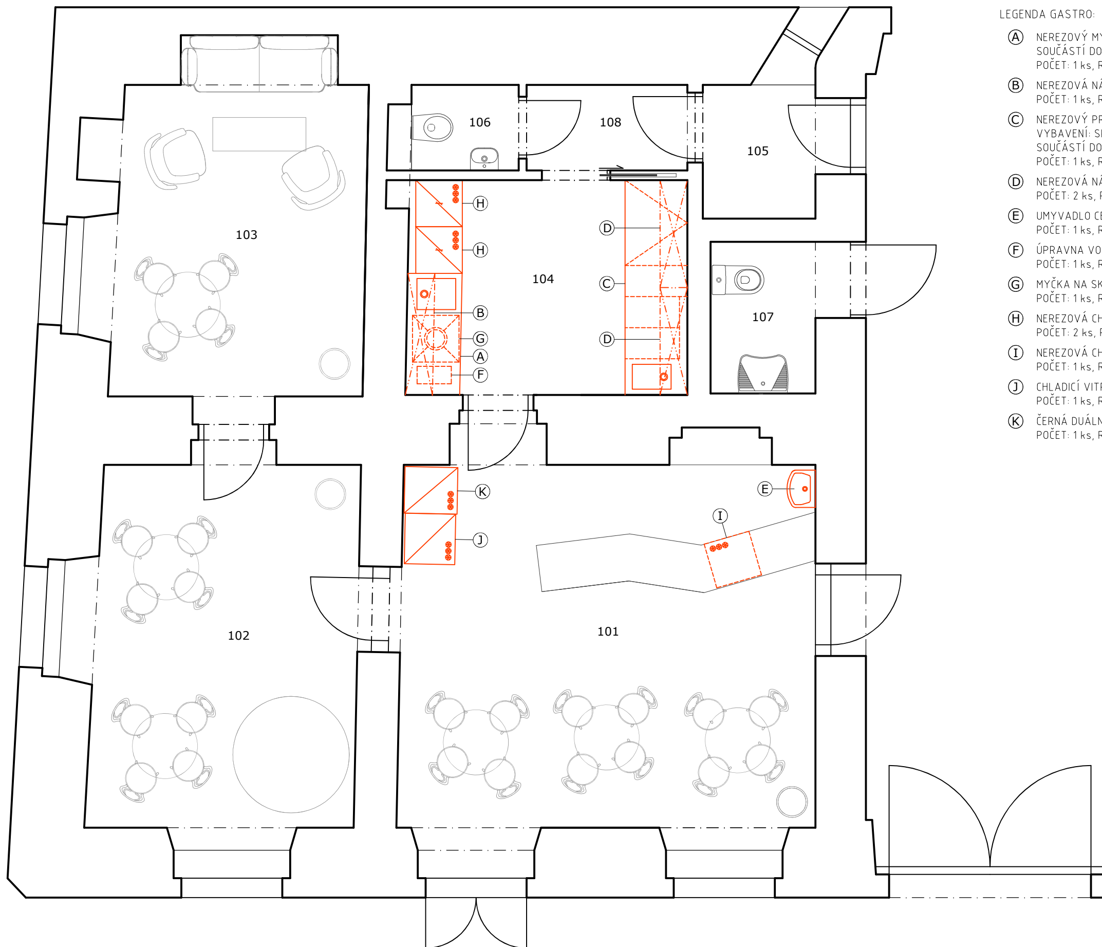
KAVÁRNA NA RADNICI - PŮDORYS 1.NP - GASTRO VYBAVENÍ NÁM. SVOBODY 823, BUČOVICE M 1:50
